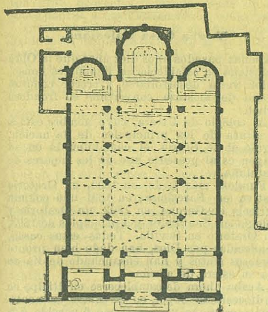
Planta de la iglesia.
